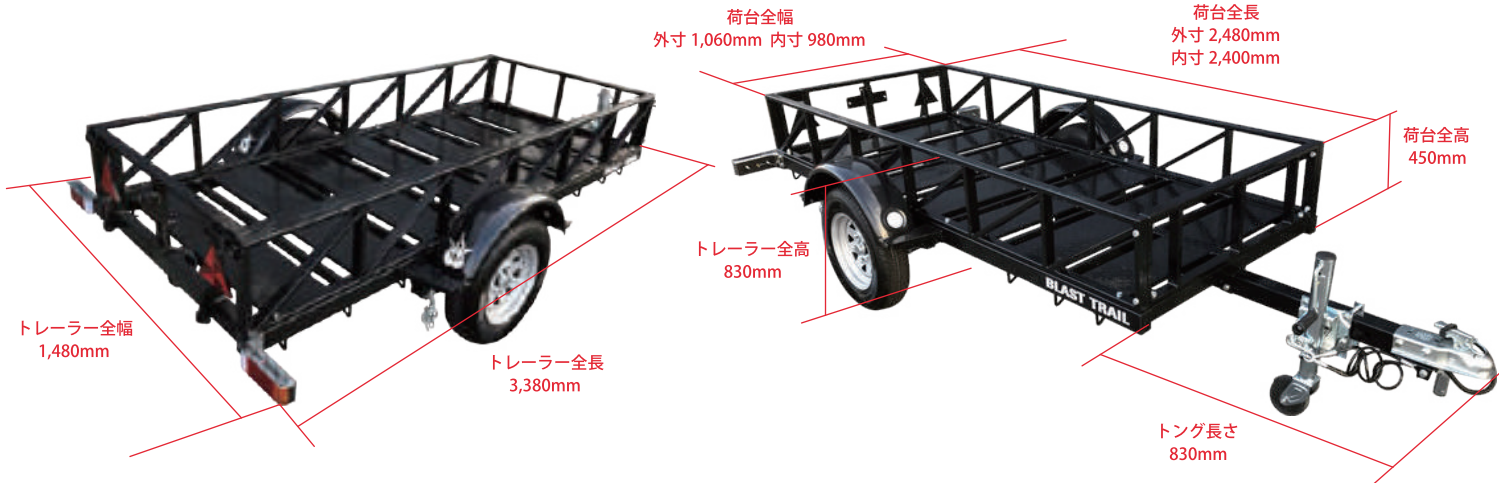
トレーラー寸法
