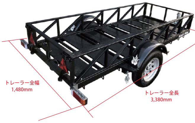
トレーラー寸法
